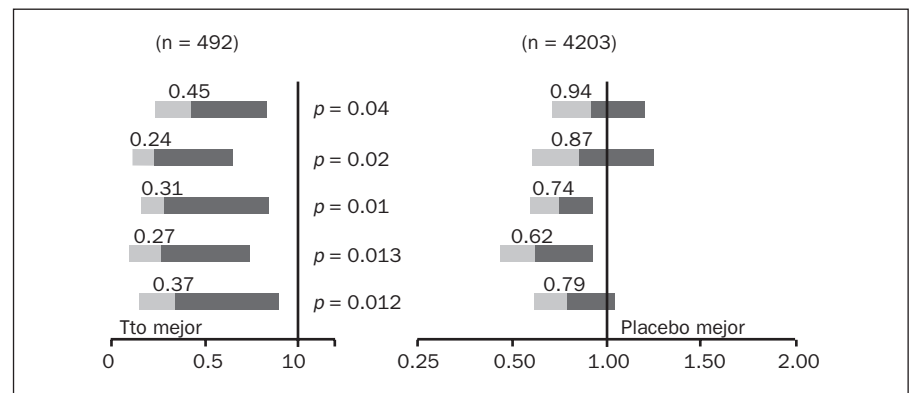
Figura 7: Efecto del control tensional obtenido en el estudio Syst-EUR (31). Comparativo entre hipertensos diabéticos no diabéticos.
